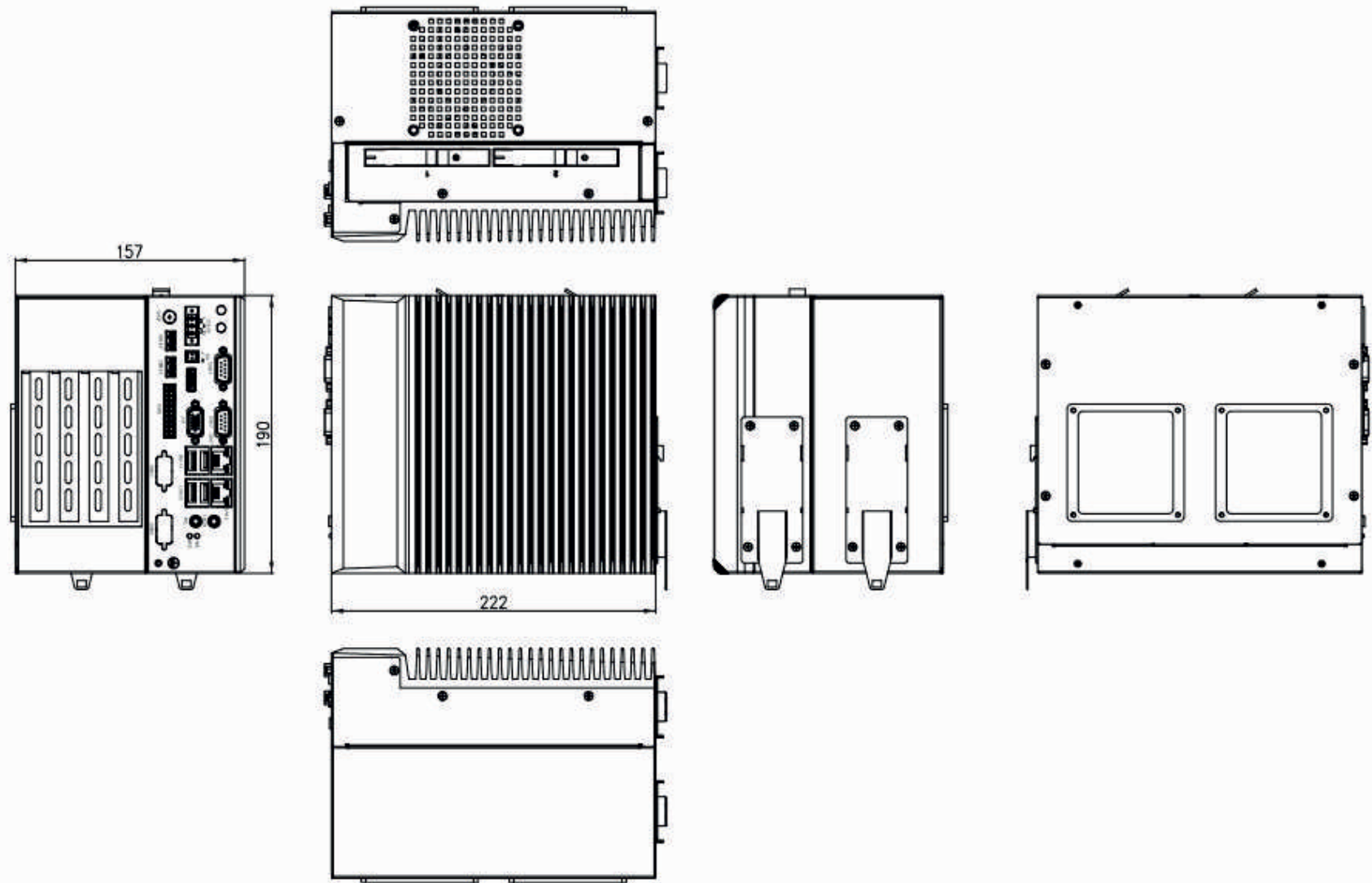
Din Rail
